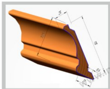
Прямиий. Довжина 2070 мм, 2550 мм
