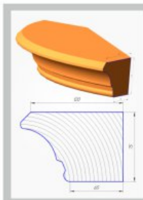
Гнугий R-300 зовнiшнiй та внутрiшнiй
